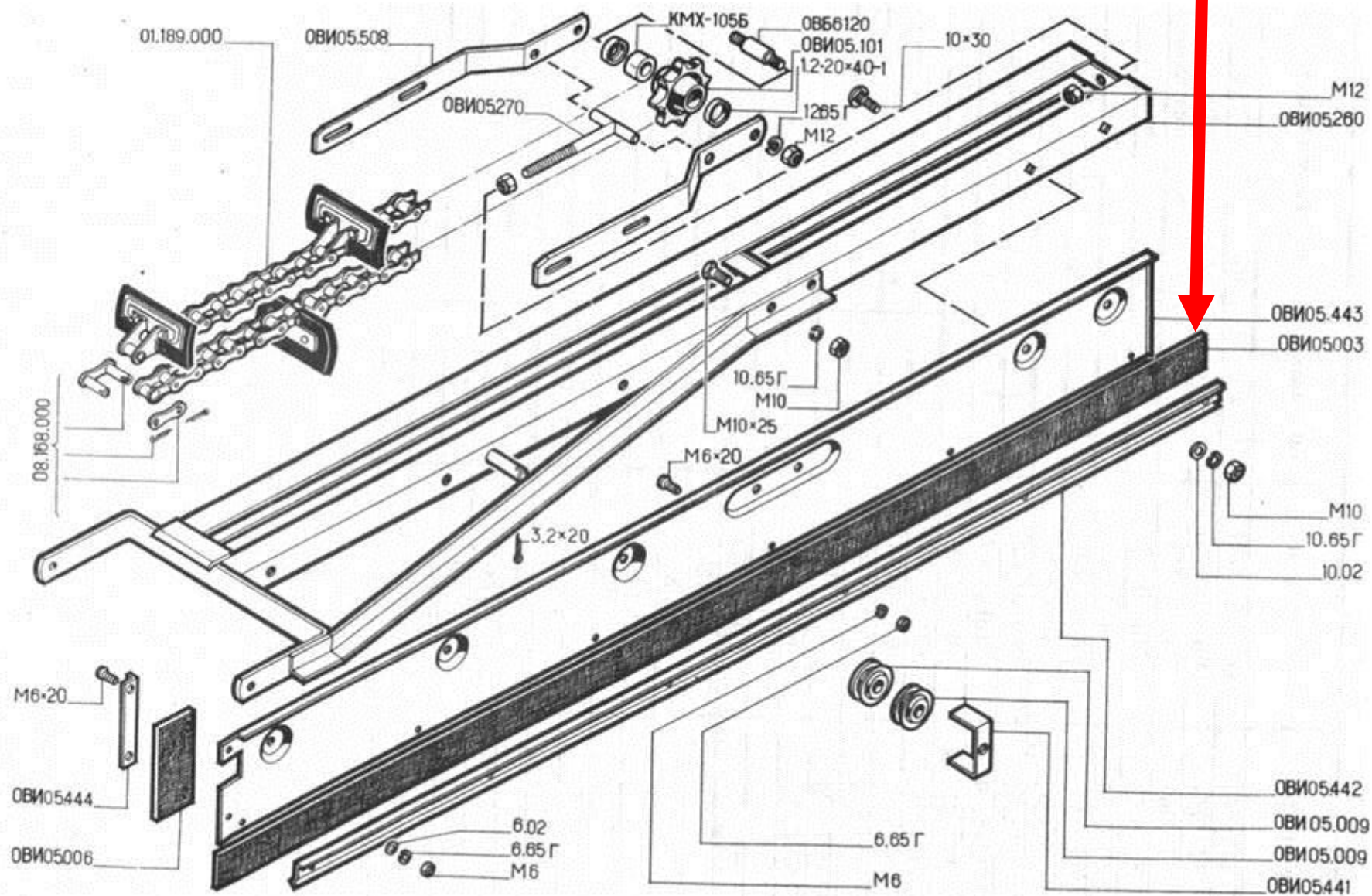
Рис. 26. Питатель ОВИ 05.200.
